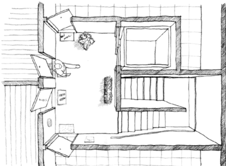
Figura 09: Um hall de prédio mais seguro com até quatro apartamentos por andar.
